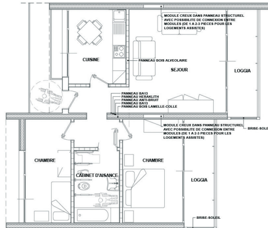
3. VUE EN PLAN - PRINCIPES TECHNOLOGIQUES - MATERIAUX
