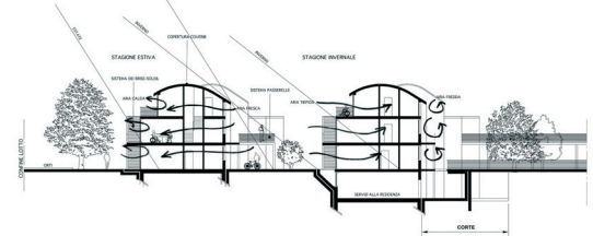
2. COUPES TRANSVERSALES - PRINCIPES BIO-CLIMATIQUES
